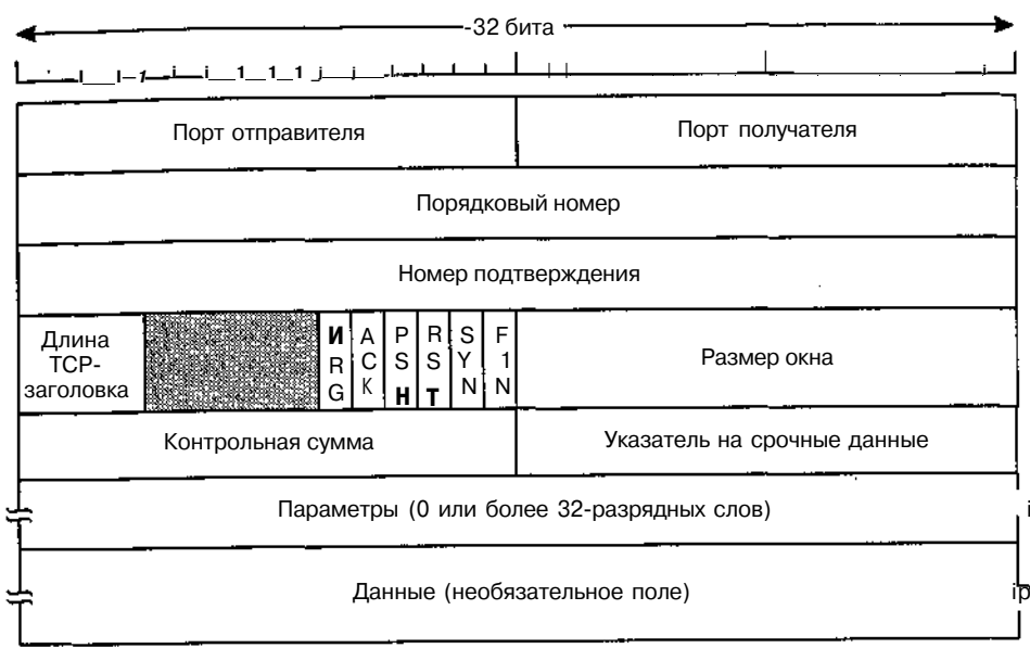
Рис. 6.23. Заголовок TCP
