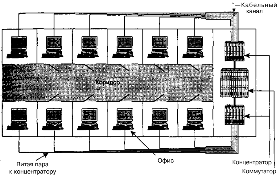
Рис. 4.44. Здание с централизованной проводкой
