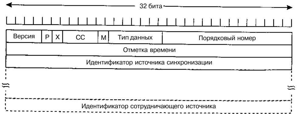
Рис. 6.21. Заголовок RTP
