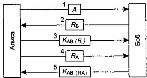
Рис. 8.28. Двусторонняя аутентификация при помощи протокола оклик—отзыв
