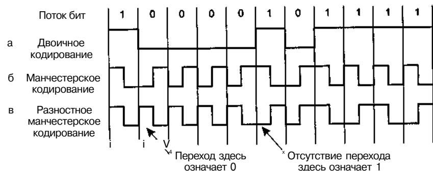
Рис. 4.15. Двоичное кодирование (а); манчестерское кодирование (б); разностное манчестерское кодирование (в)
