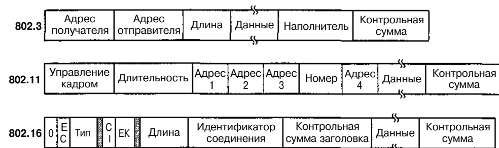
Рис. 4.37. Форматы кадров стандартов IEEE 802. Масштаб не выдержан
