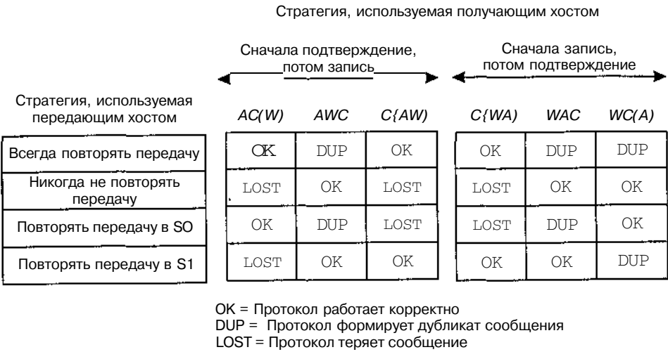
Рис. 6.15. Различные комбинации стратегий сервера и клиента
