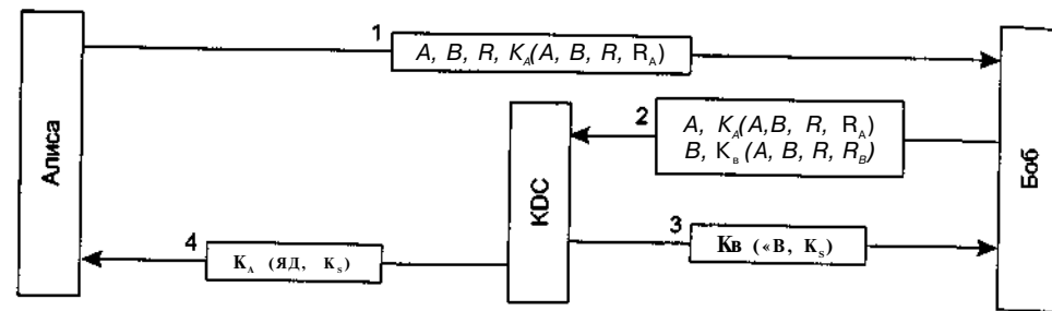
Рис. 8.37. Протокол аутентификации Отуэя—Риса (слегка упрощенный)
