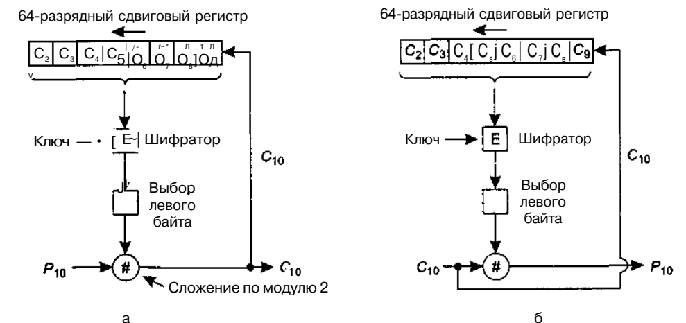
Рис. 8.11. Режим шифрованной обратной связи (а); обратная связь по выходу (б)
