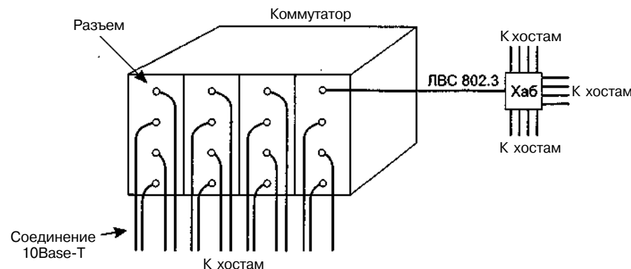
Рис. 4.19. Простой пример коммутируемой сети Ethernet
