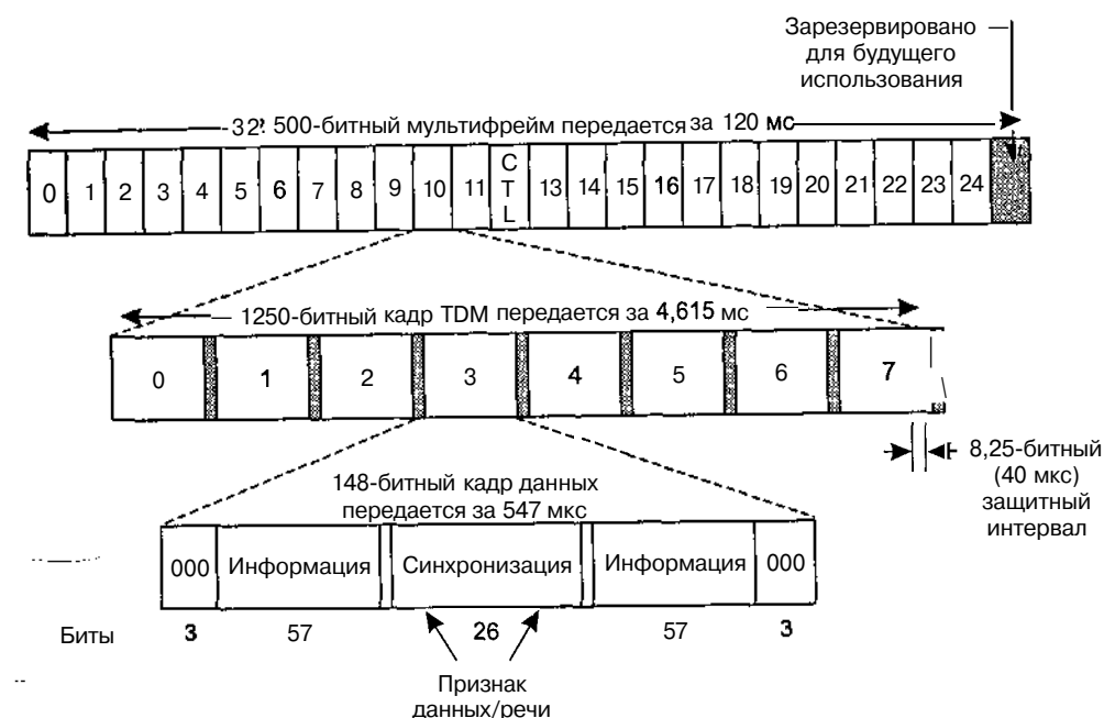
Рис. 2.38. Часть иерархической структуры кадров GSM
