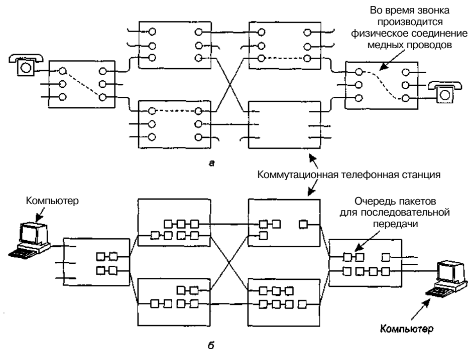
Рис. 2.33. Коммутация каналов (а); коммутация пакетов (б)
