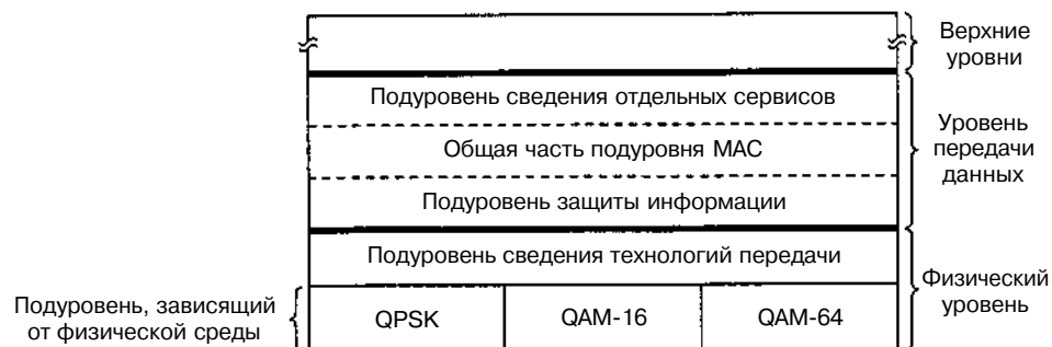
Рис. 4.28. Стек протоколов 802.16
