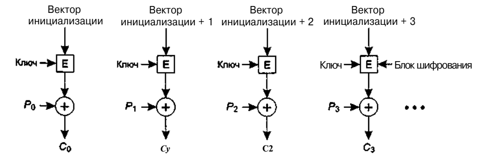
Рис. 8.13. Шифрование в режиме счетчика
