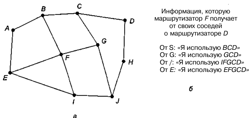
Рис. 5.57. Множество BGP-маршрутизаторов (а); информация, посланная маршрутизатору F (б)
