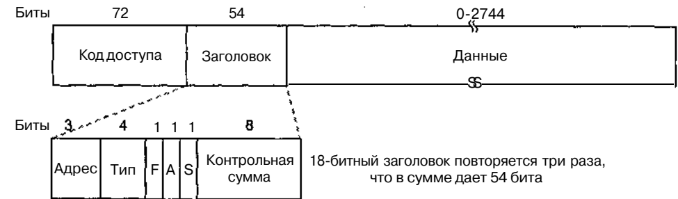
Рис. 4.34. Типичный информационный кадр Bluetooth
