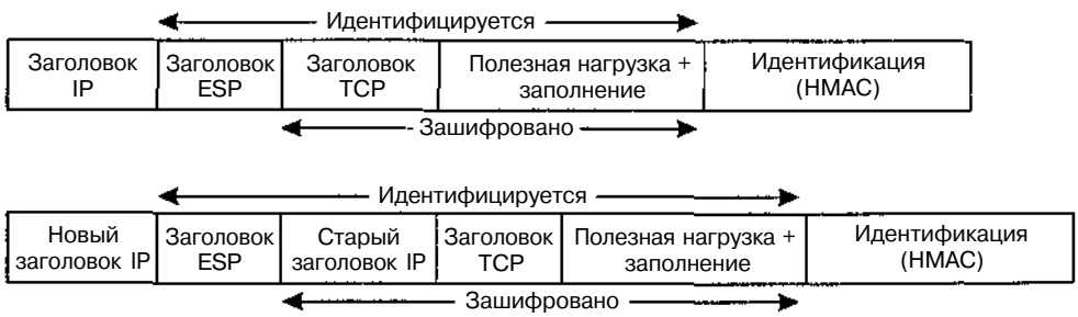
Рис. 8.24. ESP в транспортном режиме (а); ESP в режиме туннелирования (б)
