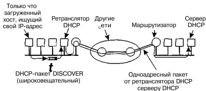
Рис. 5.54. Работа протокола DHCP
