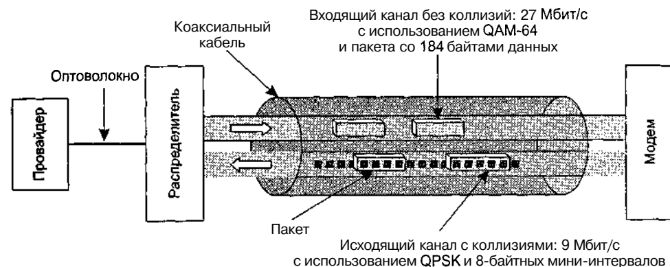
Рис. 2.43. Типичная схема входящего и исходящего каналов, принятая в США
