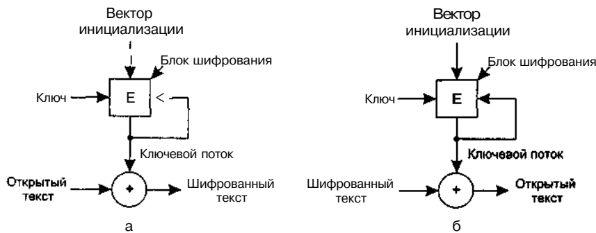
Рис. 8.12. Групповой шифр: шифрование (а); дешифрация (б)
