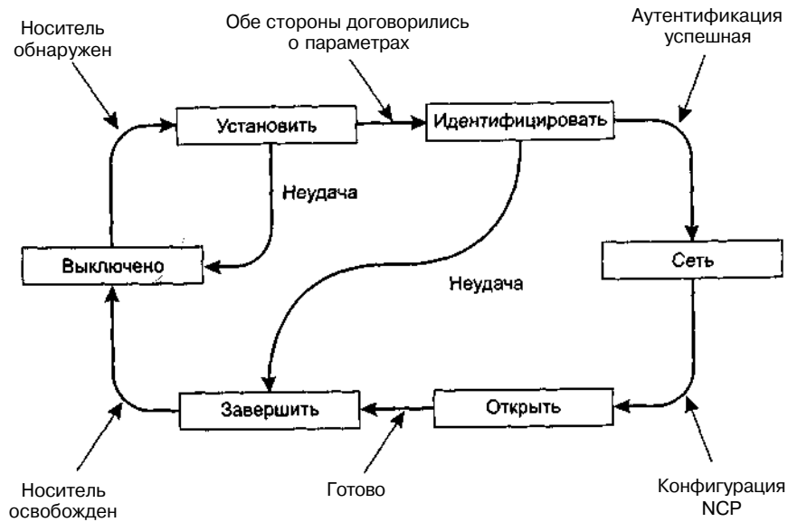
Рис. 3.21. Упрощенная фазовая диаграмма установки и разрыва соединения
