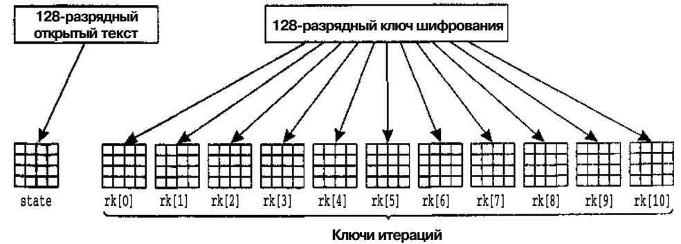
Рис. 8.8. Создание массивов state и rk
