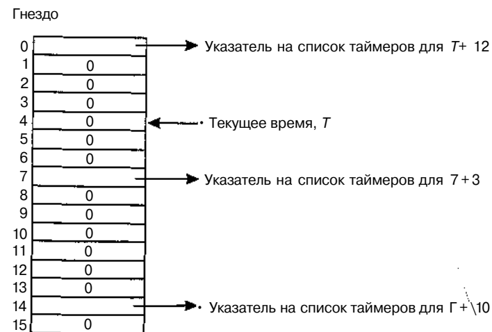
Рис. 6.39. Колесо времени
