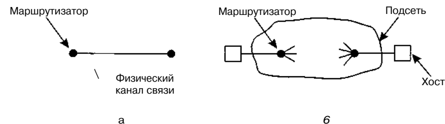
Рис. 6.4. Окружение уровня передачи данных (а); окружение транспортного уровня (б)
