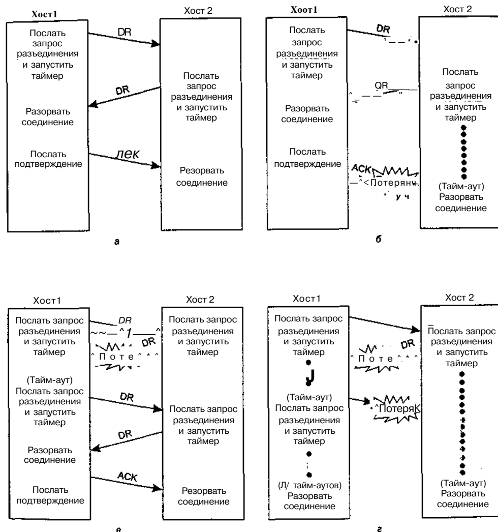
Рис. 6.11.1. Четыре сценария разрыва соединения: нормальный случай «тройного рукопожатия» (а); потеряно последнее подтверждение (б); потерян ответ (в); потерян ответ и последующие запросы (г)
