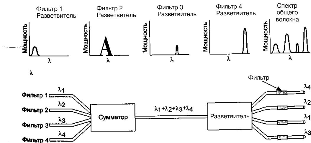
Рис. 2.28. Уплотнение с разделением длины волны
