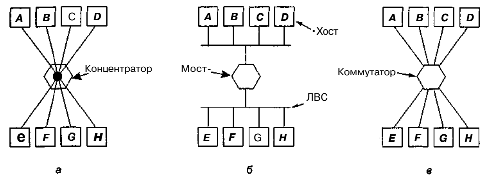
Рис. 4.43. Концентратор (а); мост (б); коммутатор (в)
