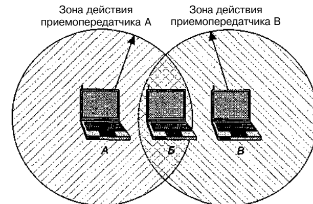
Рис. 1.32. Радиусы действия отдельных трансиверов могут не охватывать всю систему
