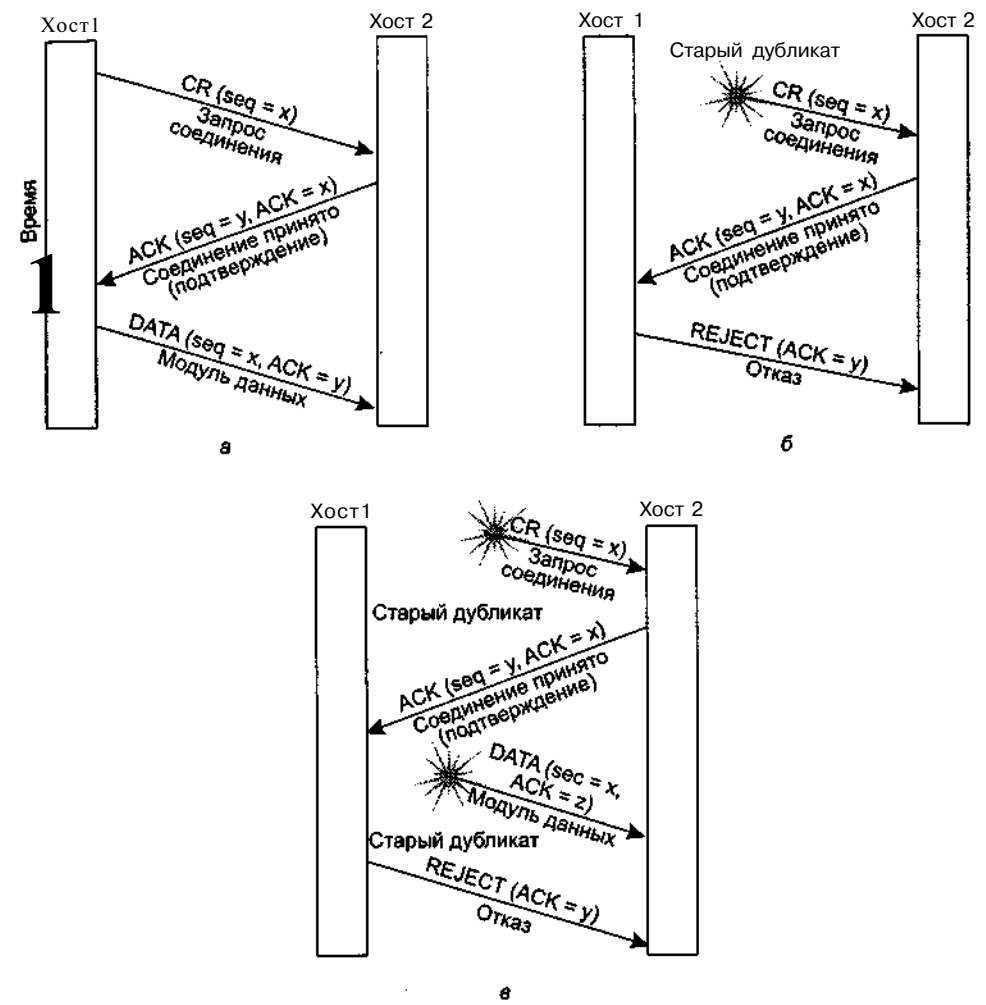
Рис. 6.8. Три сценария установки соединения с помощью «тройного рукопожатия». CR означает CONNECTION REQUEST. Нормальная работа (а); появление старого дубликата CONNECTION REQUEST (б); дубликат модуля CONNECTION REQUEST и дубликат модуля ACK (в)
