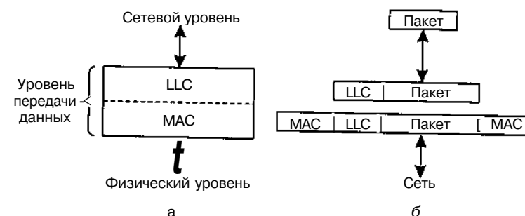
Рис. 4.21. Расположение подуровня LLC (а); форматы протокола (б)
