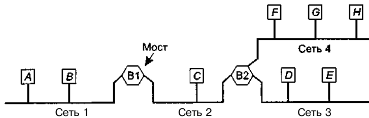
Рис. 4.38. Структура из четырех сетей и двух мостов
