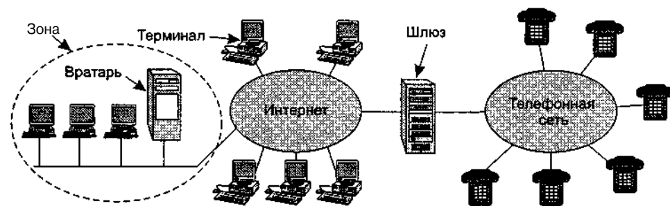
Рис. 7.32. Модель архитектуры Н.323 для интернет-телефонии
