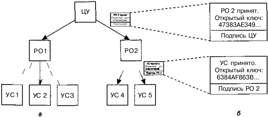
Рис. 8.22. Иерархия PKI (а); цепочка сертификатов (б)
