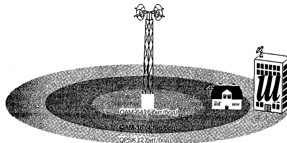
Рис. 4.29. Оперативная среда передачи данных сетей 802.16
