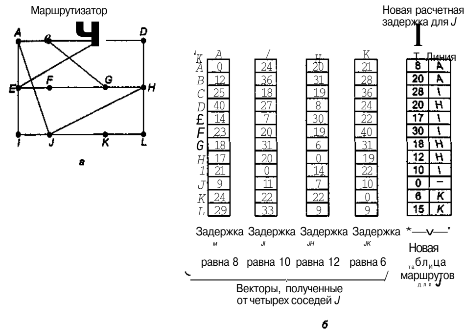
Рис. 5.7. Подсеть (а); полученные от D, I, H и K векторы и новая таблица маршрутов для J (б)
