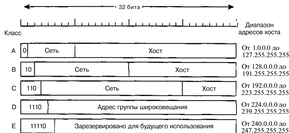
Рис. 5.48. Форматы IP-адреса
