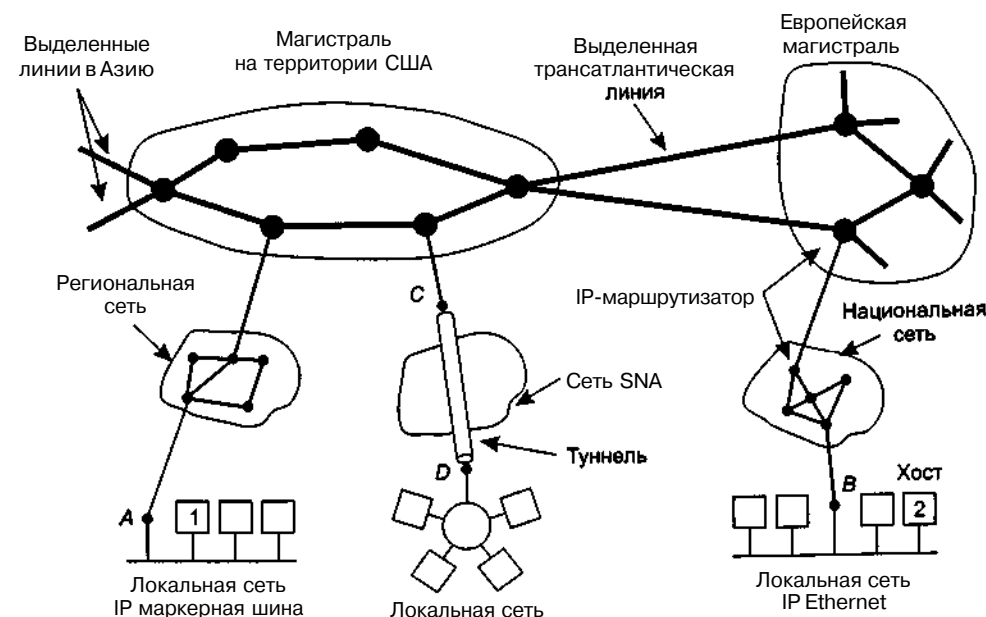
Рис. 5.46. Интернет представляет собой набор соединенных друг с другом сетей
