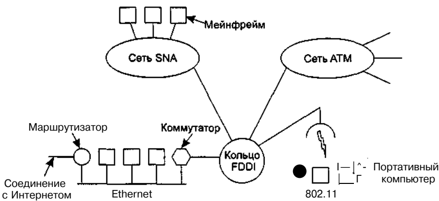
Рис. 5.37. Набор объединенных сетей
