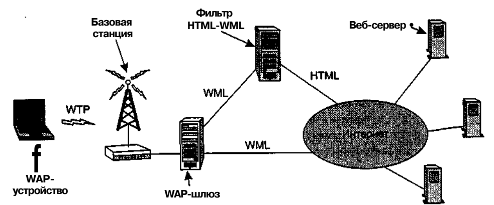
Рис. 7.21. Архитектура WAP
