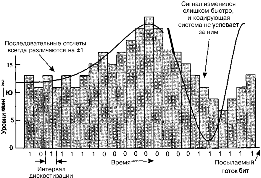
Рис. 2.30. Дельта-модуляция
