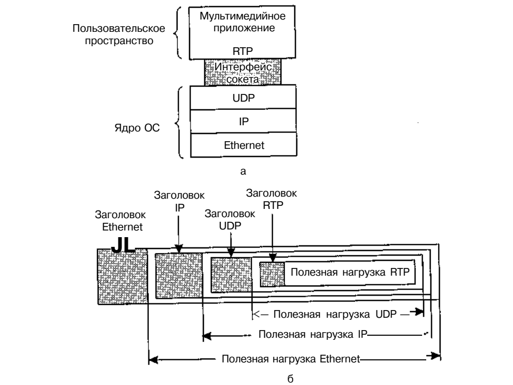
Рис. 6.20. Положение RTP в стеке протоколов (а); вложение пакетов (б)
