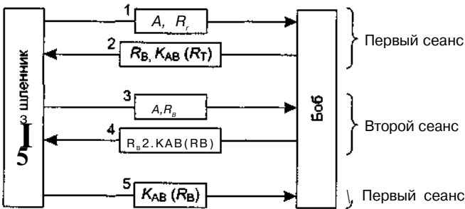
Рис. 8.30. Зеркальная атака
